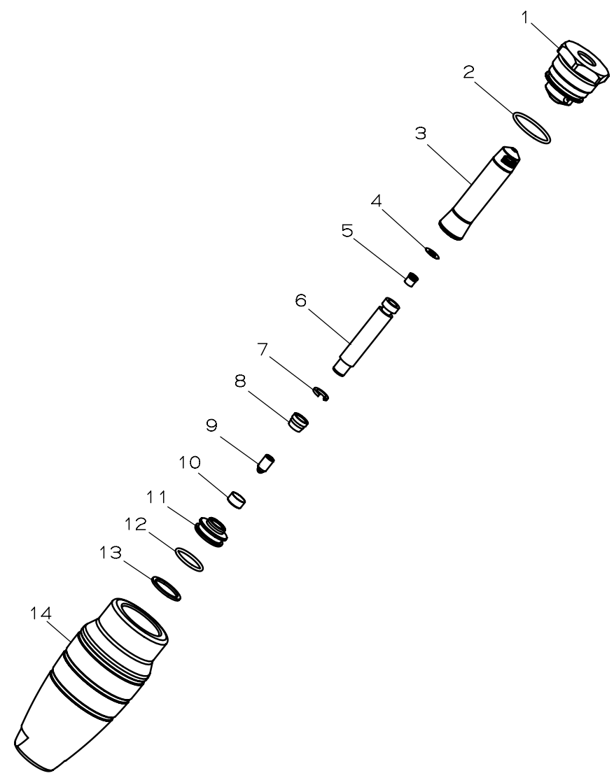
爆炸装配图 · 序号 1-14 与右侧零件清单一一对应 →
